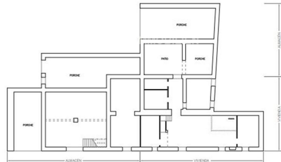
PL. 000 S.P. CONSTR. VIVIENDA 151,24 M 2 S.P. CONSTR. ALMACÉN 142 M 2 S.P. CONSTR. PARKING 20,50 M 2 S.P. CONSTR. TOTAL VIVIENDA 151,24 M 2 S.P. CONSTR. TOTAL ALMACÉN 142 M 2 S.P. CONSTR. TOTAL PARKING 20,50 M 2
